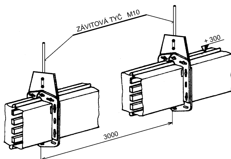
Upevnění PPR na závitovou tyč
