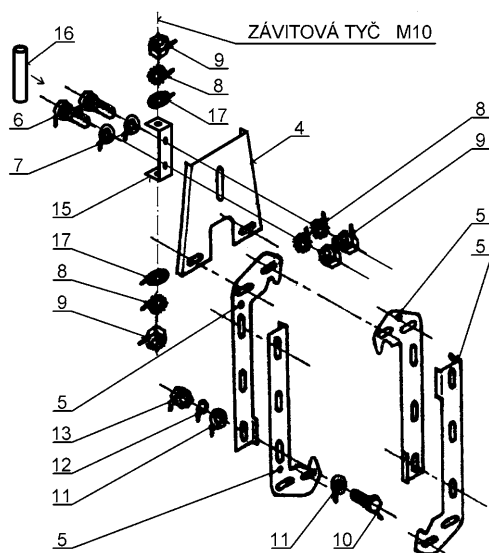
Sada upevňovacích dílců a součástí pro upevnění na závitovou tyč ST
