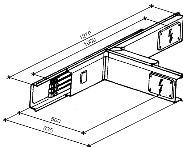
Odbočný dílec horizontální OH
