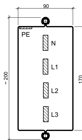
Provedení 3+N+PE (250–315 A)
