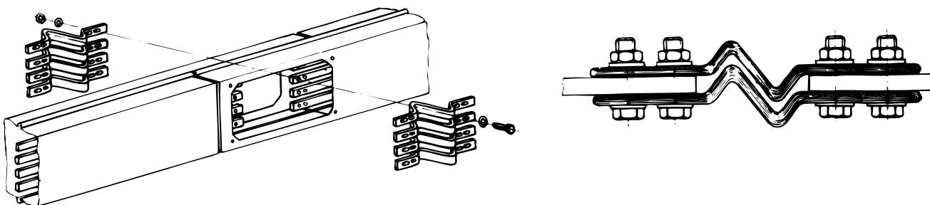
Příklad použití a sestavení pružných dilatačních spojek v prostoru navazujících dílců
