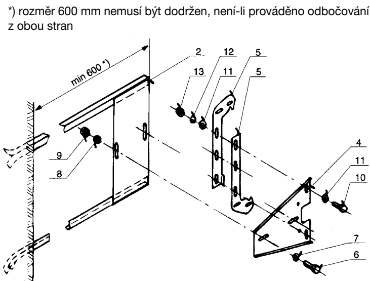
Sada upevňovacích dílců a součástí pro upevnění PPR na výložníky SV 1)
